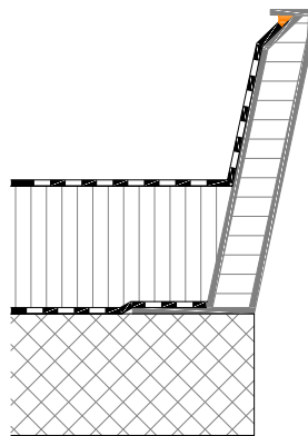
Anschluss mit Kunststoffdichtungsbahn
