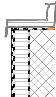
Anschluss bituminös oder mit Kunststoffdichtungsbahn
