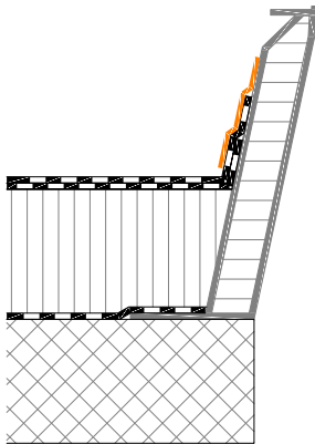
Anschluss bituminös mit zusätzlichem Flüssigkunststoffabschluss
