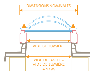
MINI-CHÂSSIS EN POLYESTER * Hauteur: 15 cm
