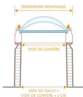
CHÂSSIS VERTICAL EN POLYESTER * Hauteurs: 15/30/50 cm
