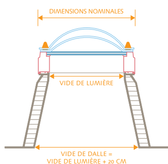
CHÂSSIS CONIQUE EN POLYESTER * Hauteurs: 15/30/50 cm
